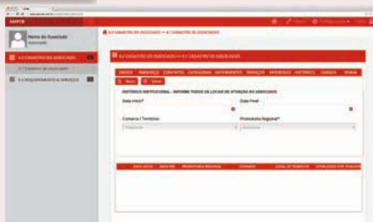
Tela 9 - Para inserir informações sobre sua vida funcional (comarcas e promotorias em que atuou ou atua), clique na aba “Histórico”. Atualize as informações e clique em “Salvar”.
